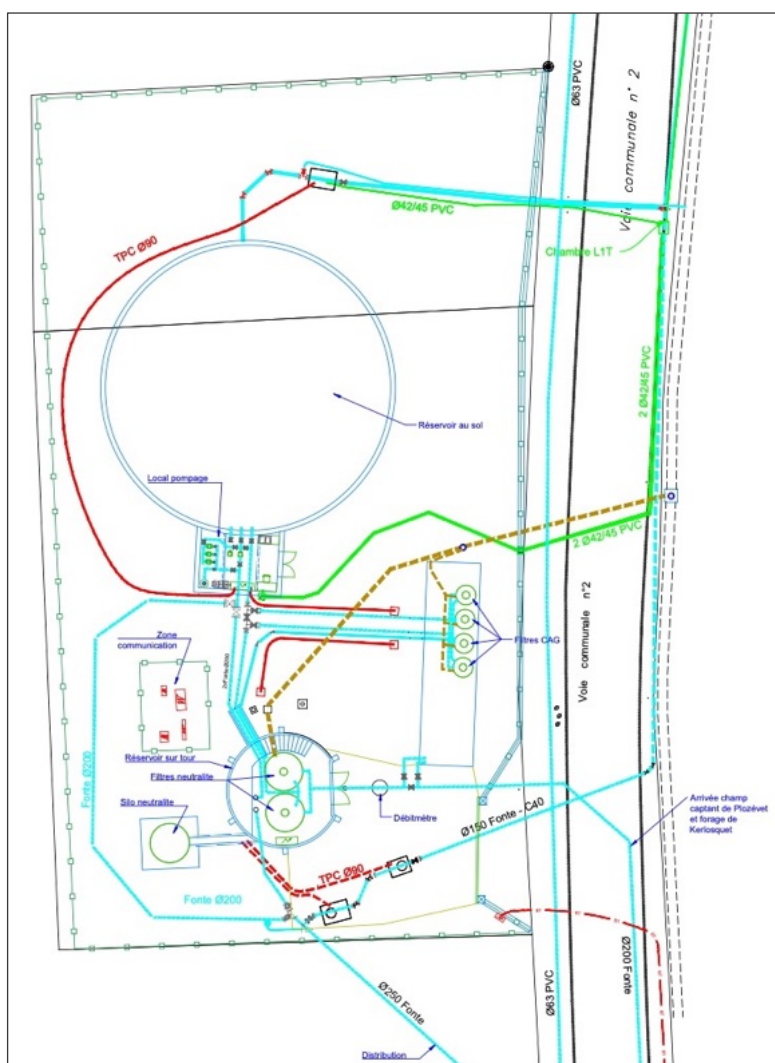
Plan actuel de l'usine de traitement avant travaux
